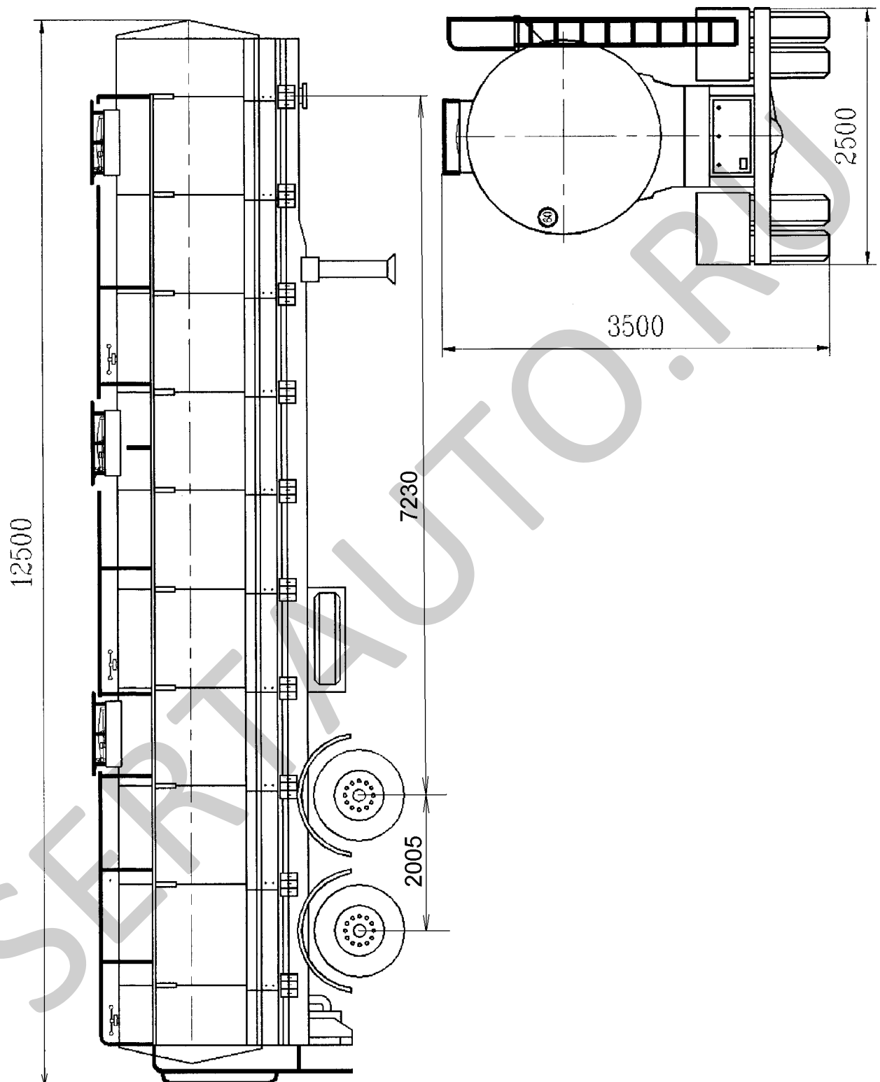
Рис.3. Полуприцеп-цистерна модели 963432 (96343-0000010-20) / Г6-ОПА-9908 на шасси СЗАП 9908
