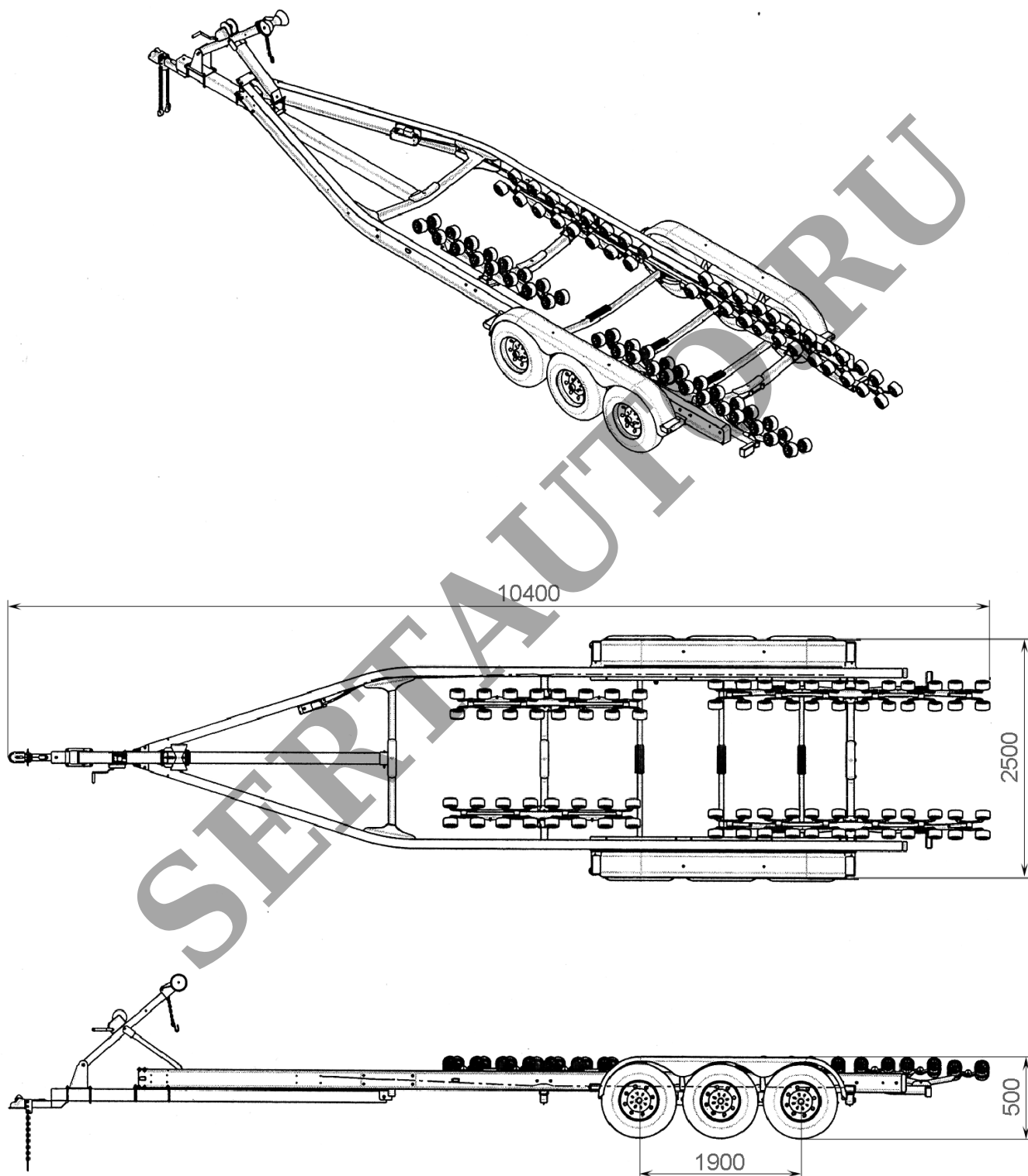
Прицеп SL150ALUM для перевозки катера (лодки)
