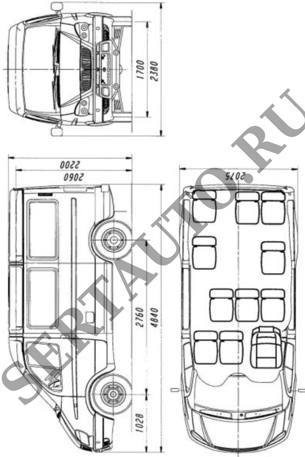
Автобус 32871D (32871-0000010-03)
