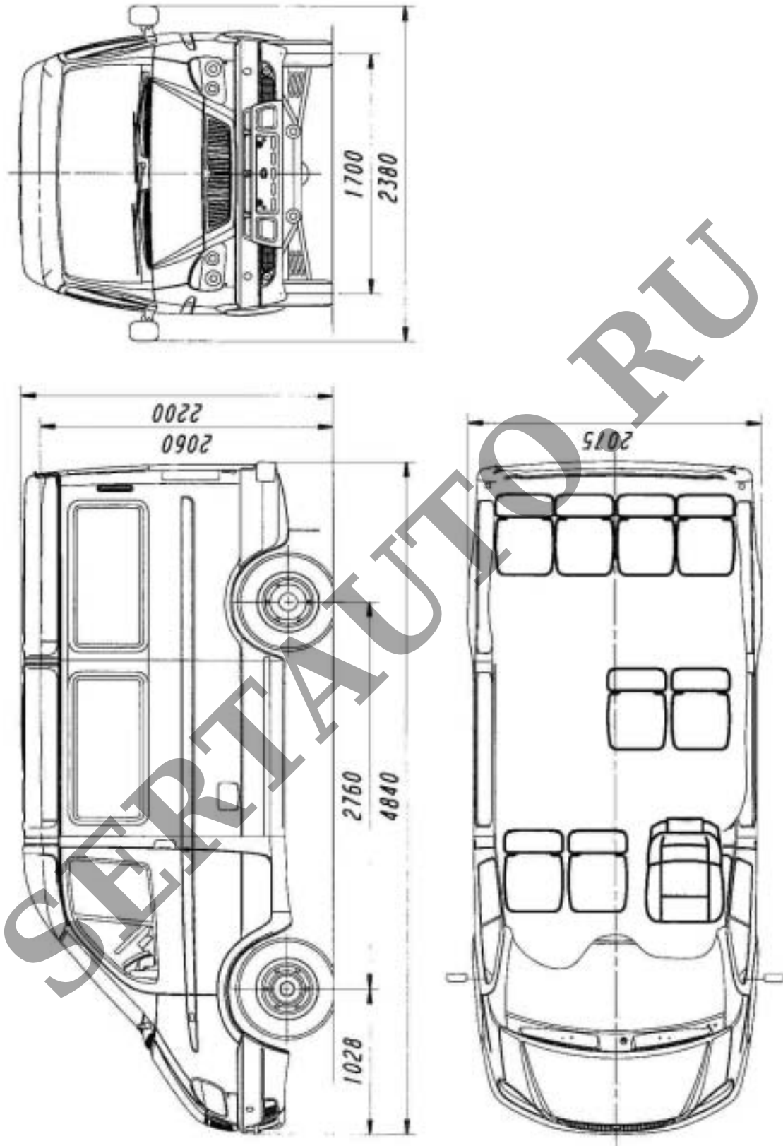
Автобус 32871В (32871-0000010-02)
