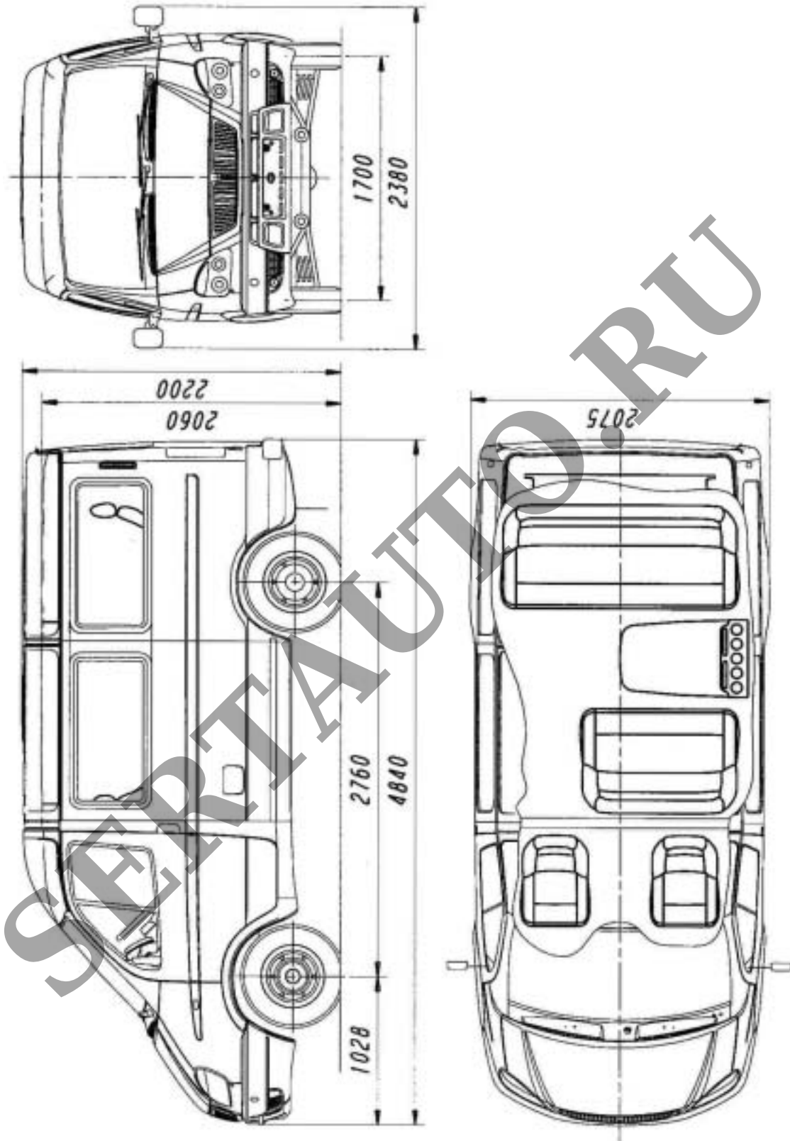
Автобус 328710 (32871-0000010)
