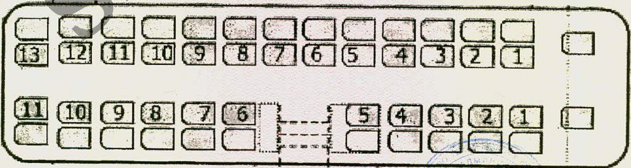
Планировка автобуса Mercedes-Benz типа Travego 15 RHD (48 + 1(сидение водителя) + 0...1 (экипаж))
